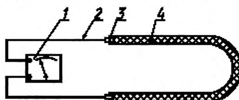
1 — измерительный прибор; 2 — проводник; 3 — электрод; 4 — рукав
