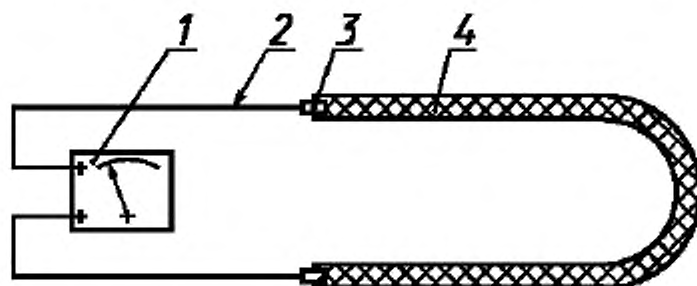
1 — измерительный прибор; 2 — проводник; 3 — электрод; 4 — рукав
